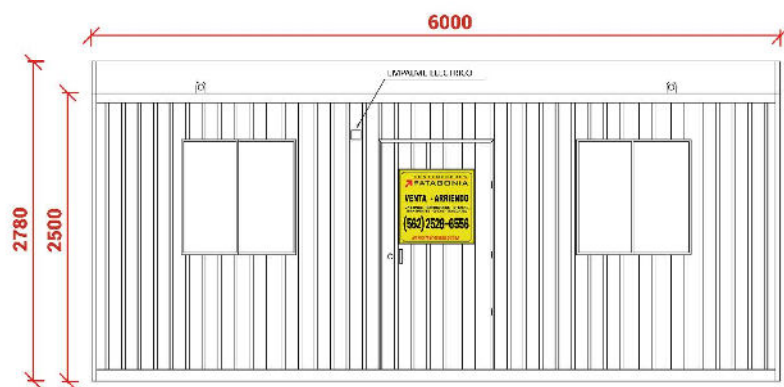
Elevación Sur
