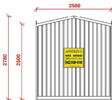
Elevación Este
