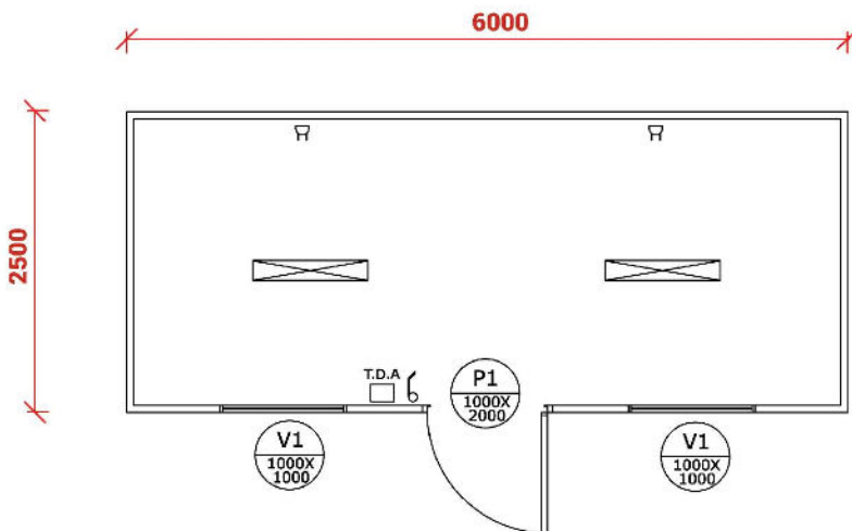
Planta
