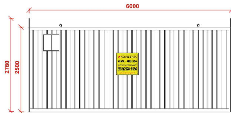
Elevación Norte
