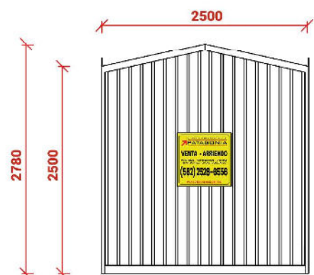
Elevación Este
