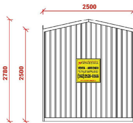
Elevación Este
