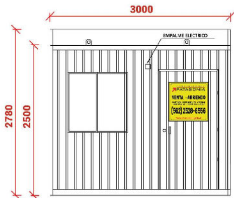
Elevación Sur
