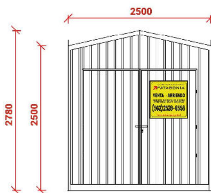
Elevación Este
