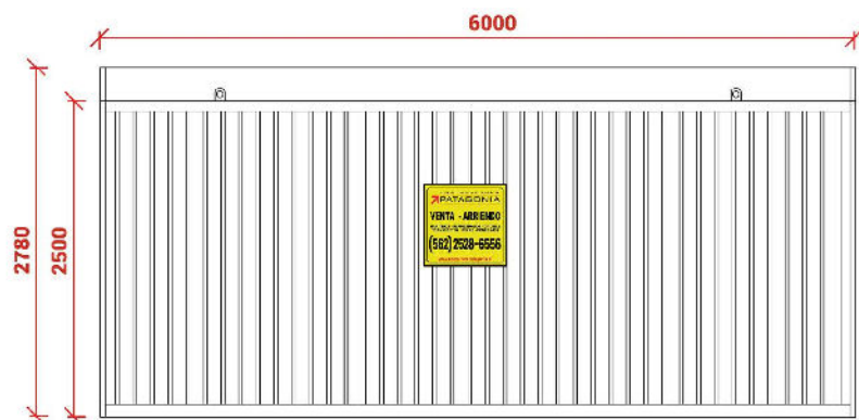
Elevación Sur
