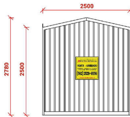
Elevación Oeste
