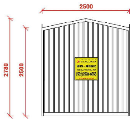
Elevación Oeste
