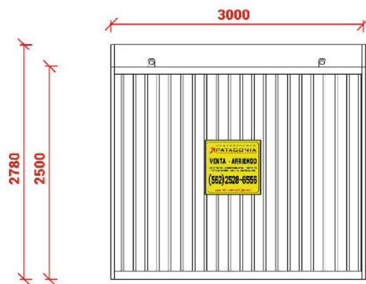
Elevación Norte
