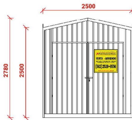
Elevación Este
