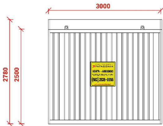
Elevación Sur
