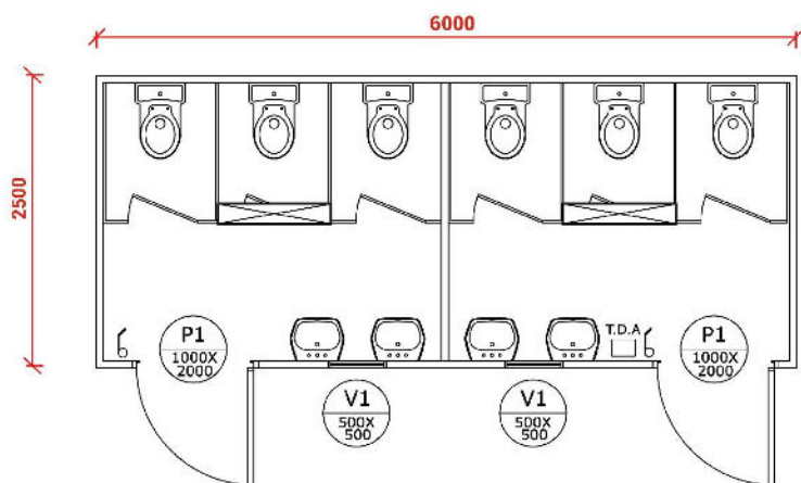
Planta
