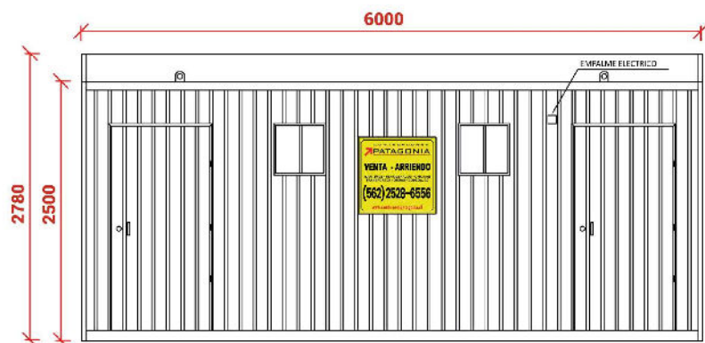
Elevación Sur
