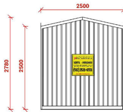
Elevación Oeste
