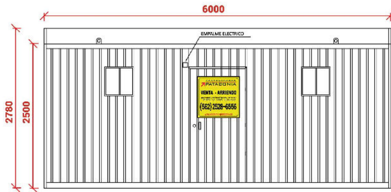
Elevación Sur
