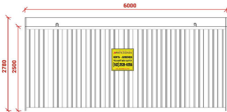
Elevación Norte
